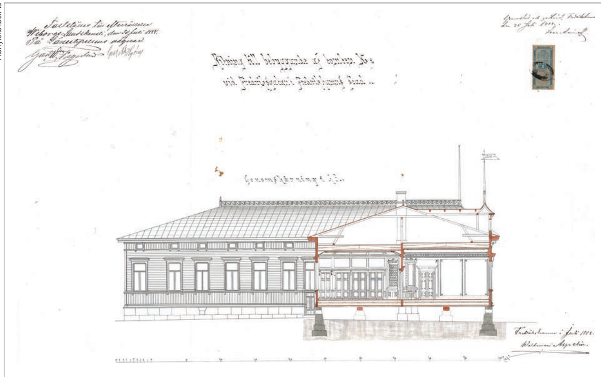
Arkkitehti W. Aspelinin laatima julkisivuleikkauspiirros pääsalien kohdalta Aladinin kaupunkipalatsista vuodelta 1888.
