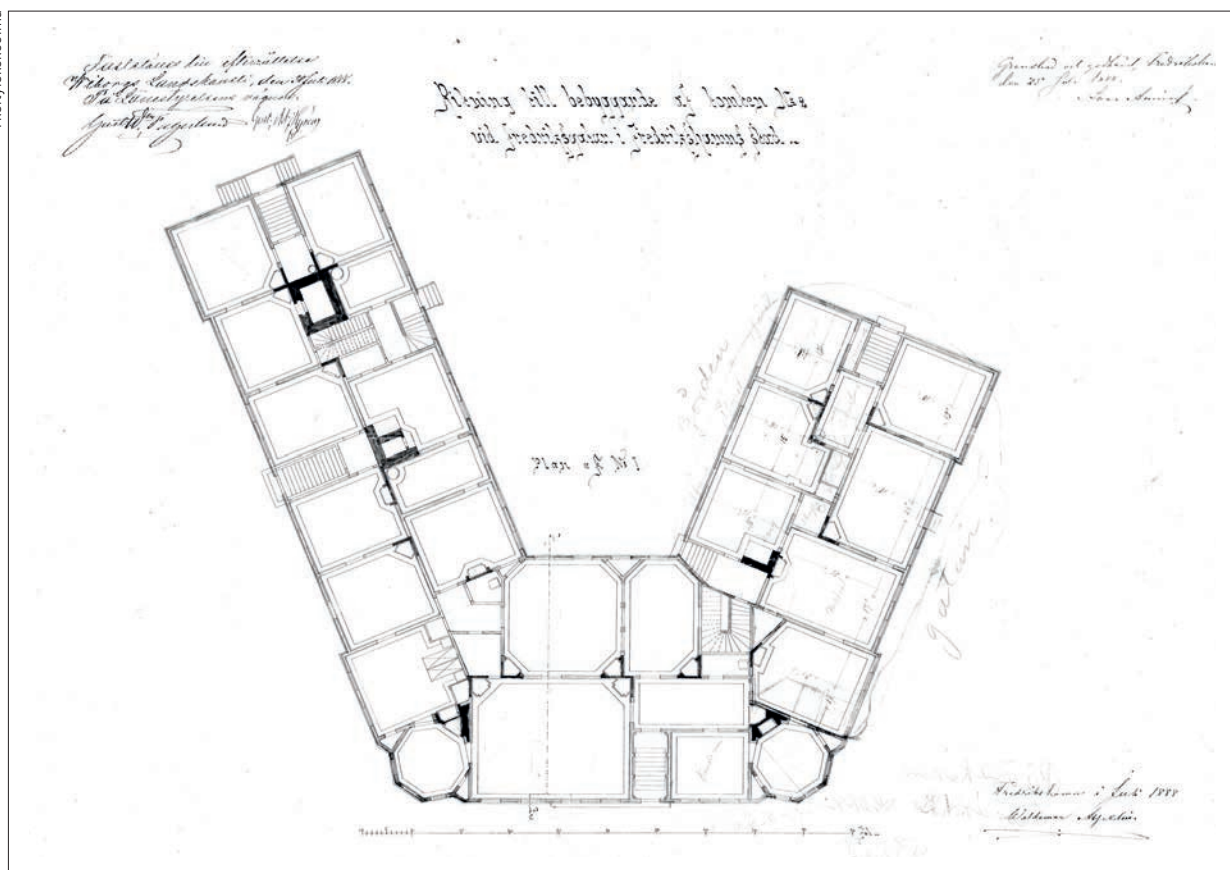
Arkkitehti W. Aspelinin laatima pohjapiirros Aladinin kaupunkipalatsista vuodelta 1888.
