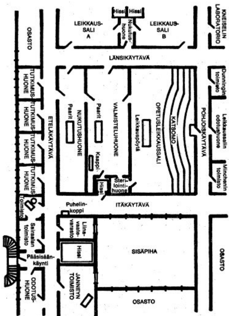
Hollantilaisen sairaalan pohjapiirros
