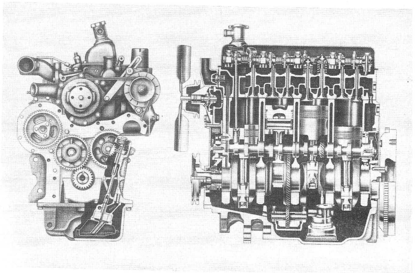
Kuva 3 4-sylinterinen dieselmoottori
