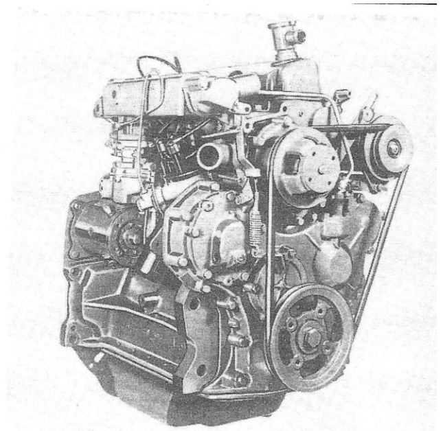
Kuva 2 Bensiinimoottori
